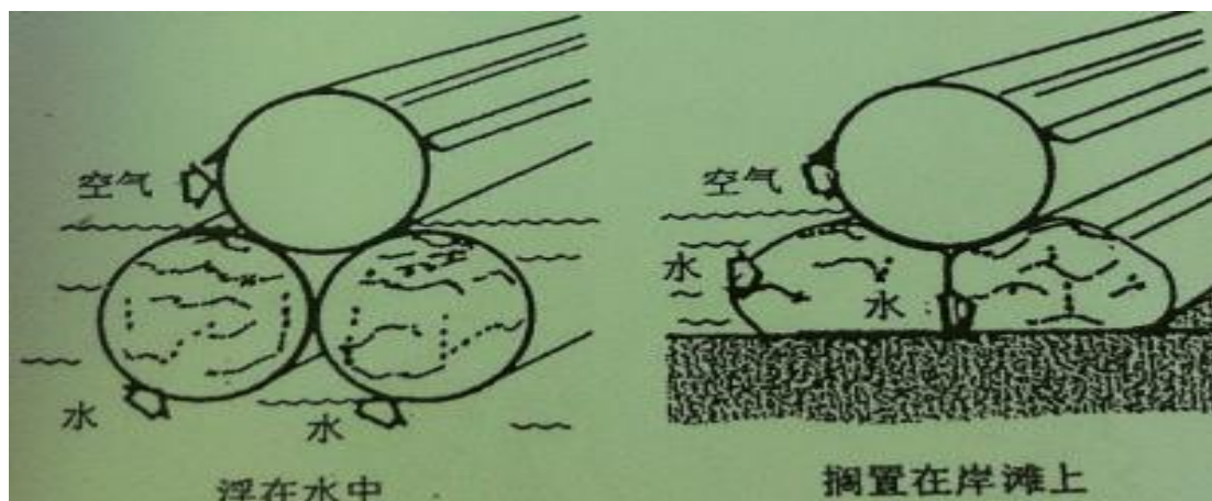
图 4-3 拦截围栏
