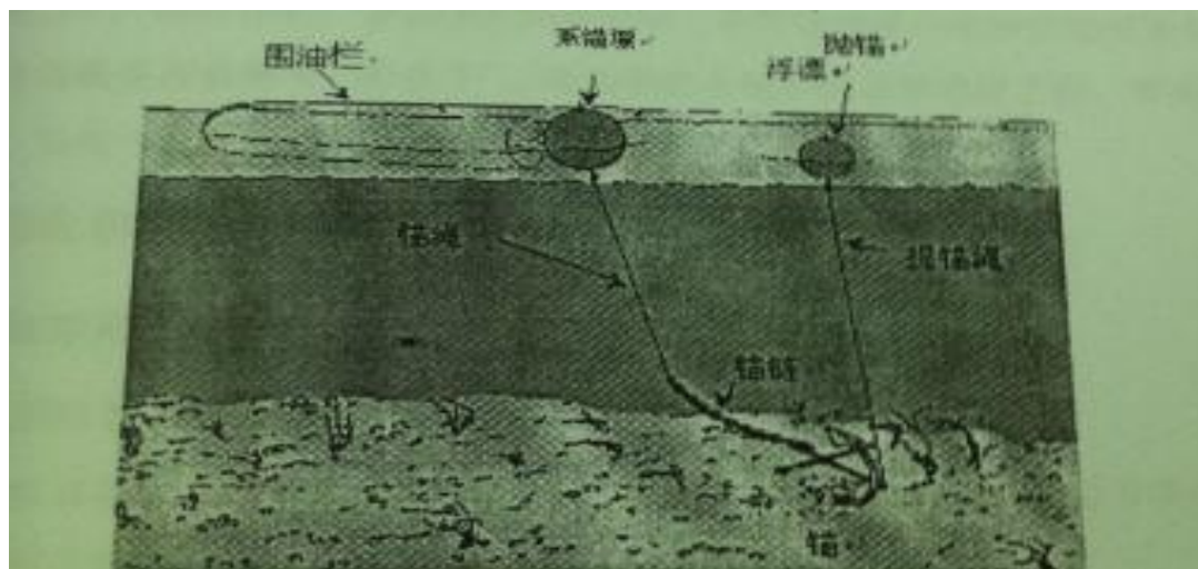
图 5-5 围油栏用锚的布放形式
