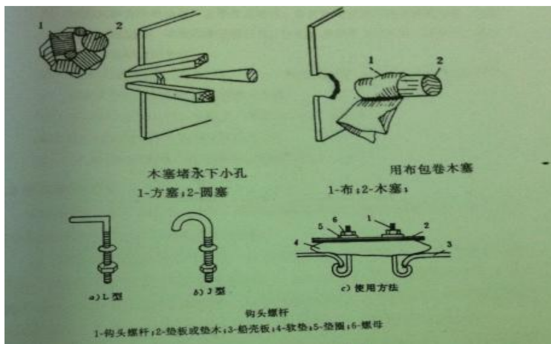
图 3-1 水线以上破口应急堵漏示意图
