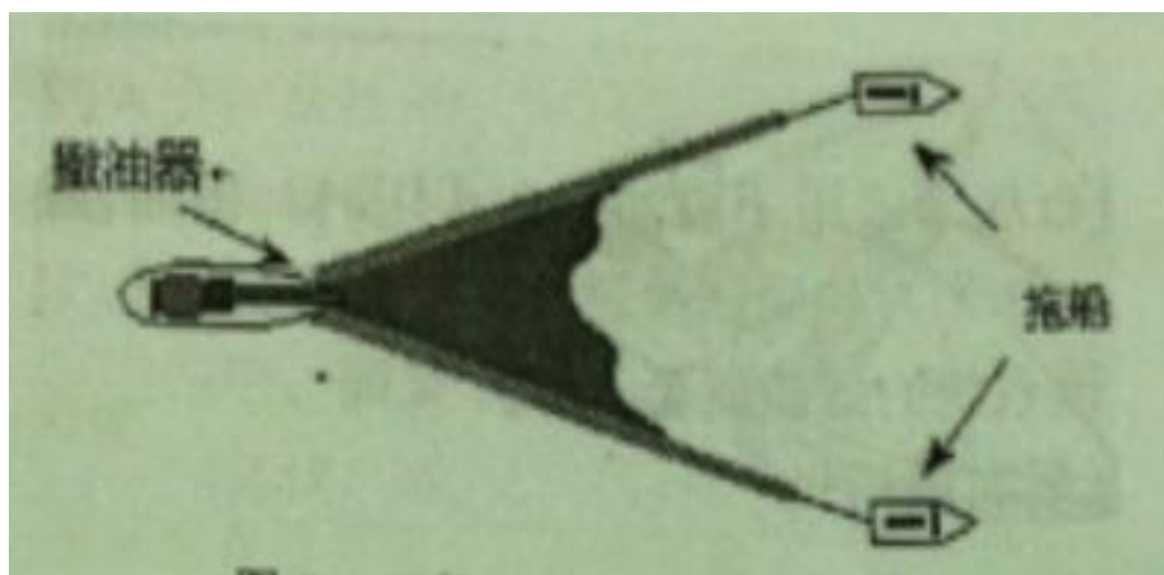
图 5-4 三船开口 U 形布放围油栏
