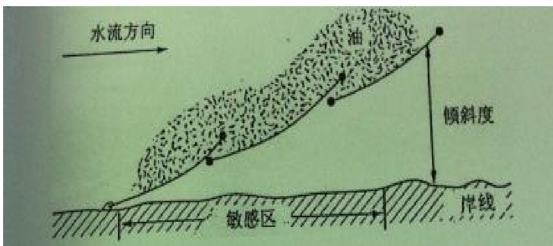
图 4-2 转移围栏
